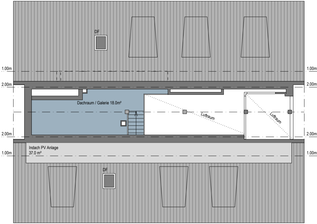
2. DACHGESCHOSS
