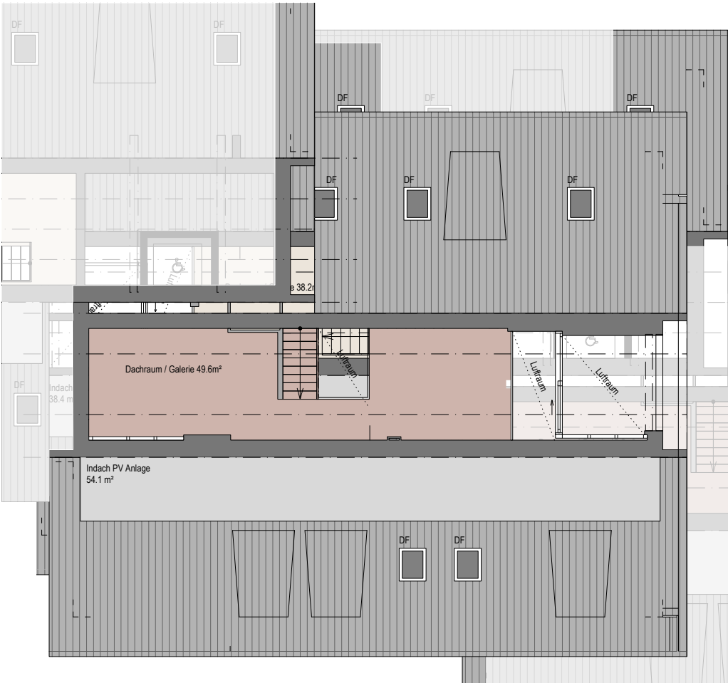
2. DACHGESCHOSS
