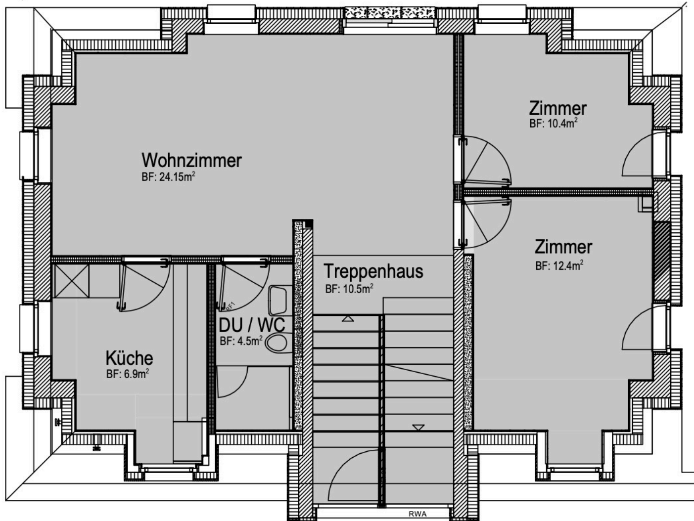
Grundriss DG
