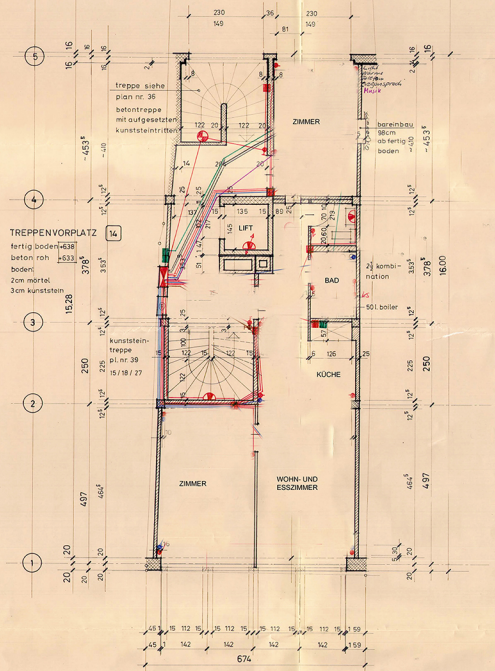
2. OBERGESCHOSS
