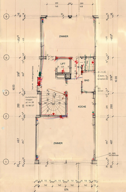
3+4. OBERGESCHOSS
