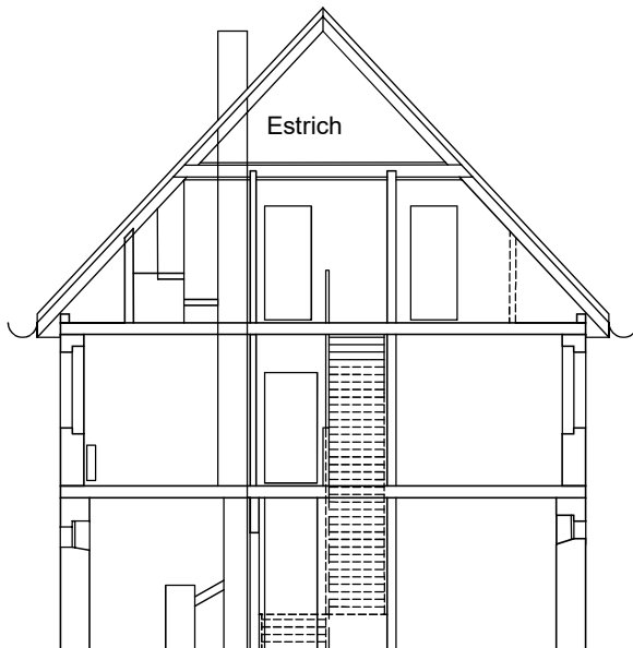
Schnitt1-1
