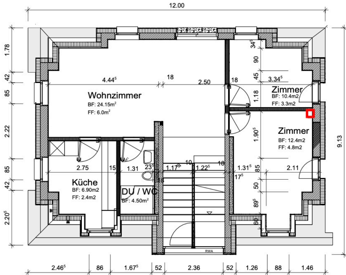
Grundriss DG
