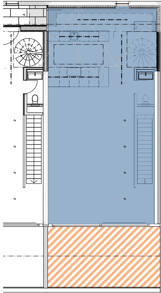
Grundriss 4. Obergeschoss Brutto Wohnfläche: 85.3m 2 Aussenfläche: 25.7m 2
