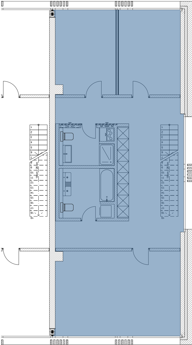
Grundriss 3. Obergeschoss Brutto Wohnfläche: 109.5m 2
