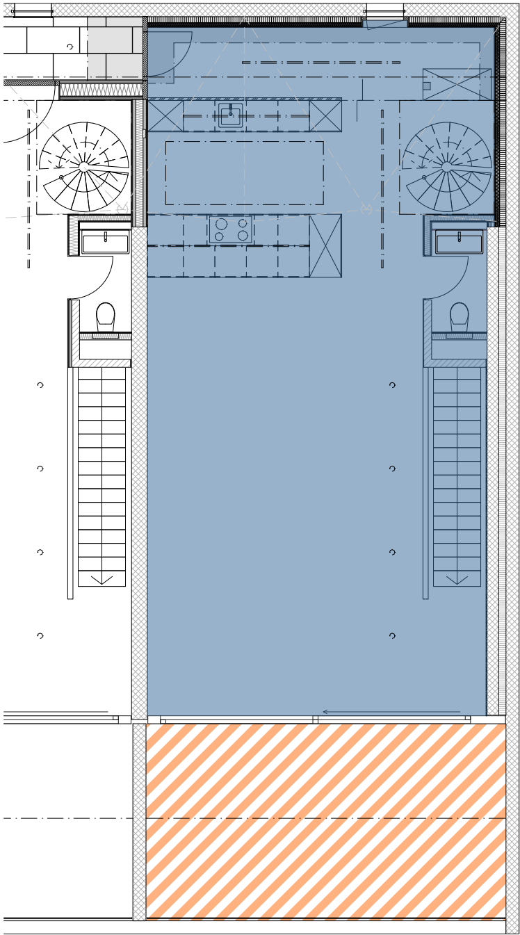
Grundriss 4. Obergeschoss Brutto Wohnfläche: 85.3m 2 Aussenfläche: 25.7m 2
