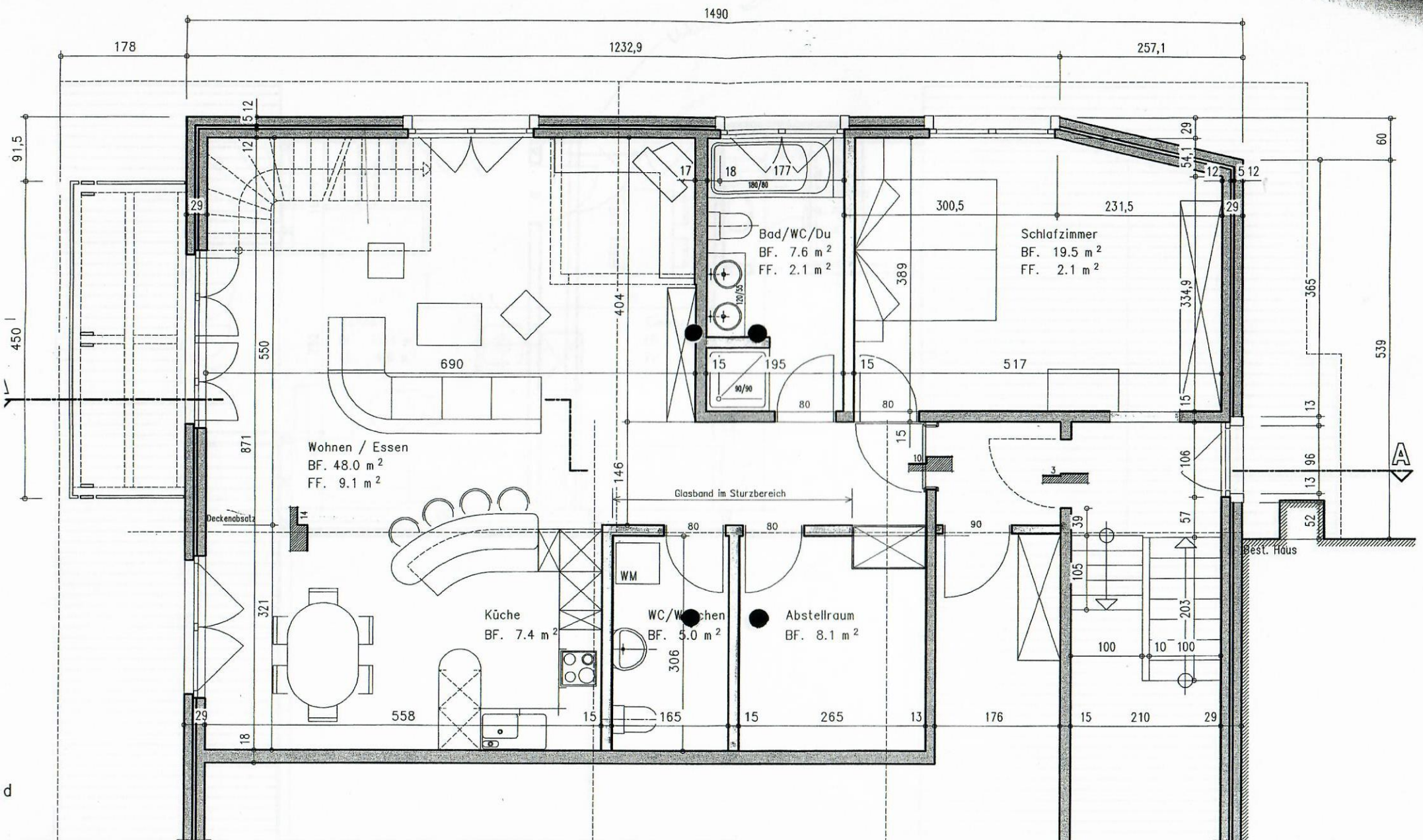
GRUNDRISS OBERGESCHOSS
