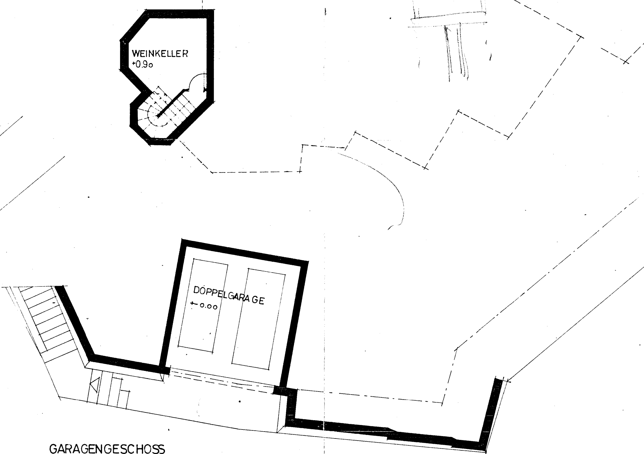
GARAGENGESCHOSS
