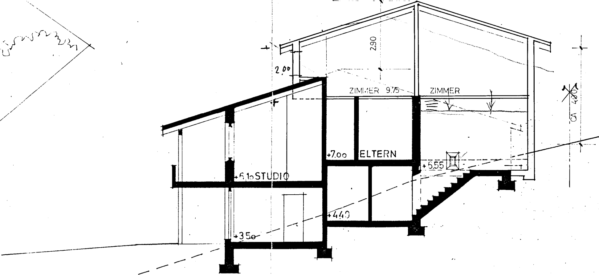
SCHNITT A-A
