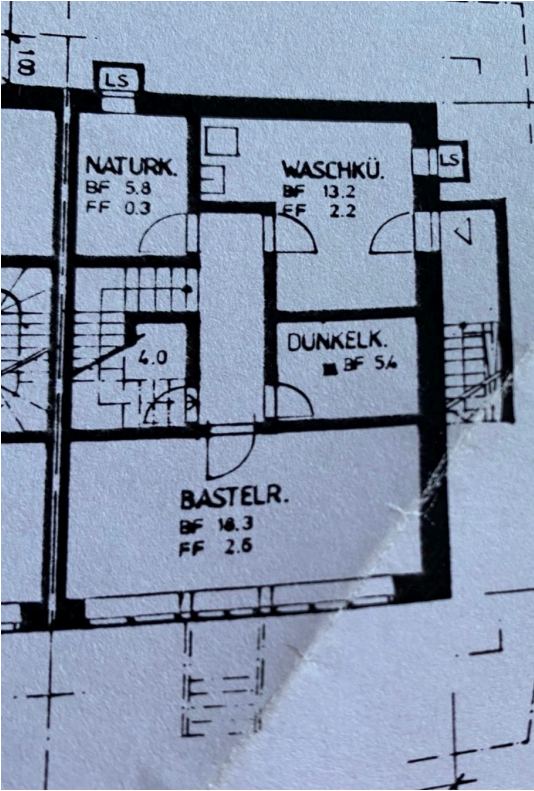
UG (Keller)
