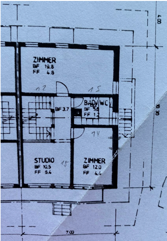
1. OG
