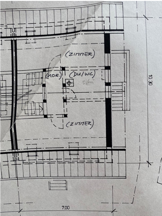
2. OG
