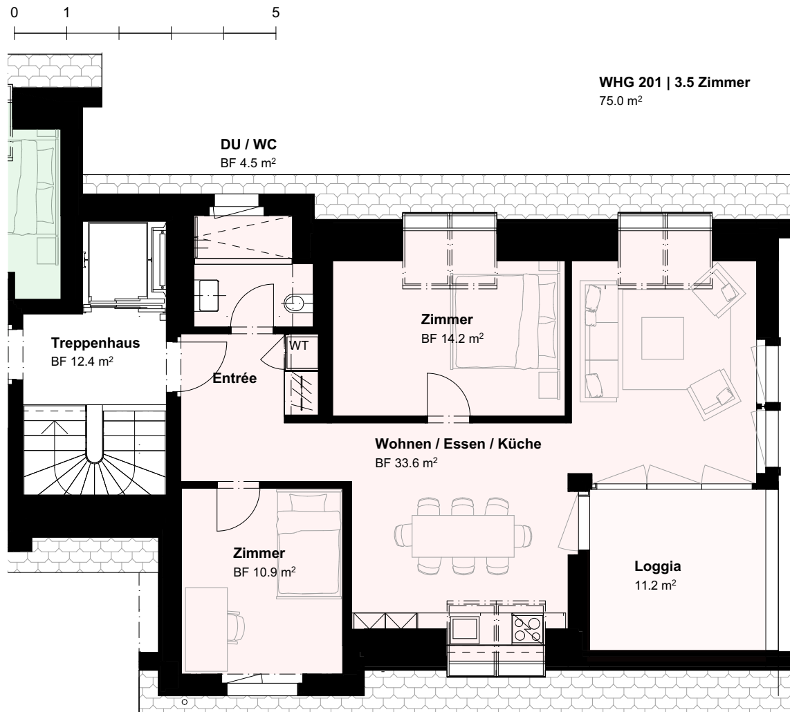
Grundriss Dachgeschoss
