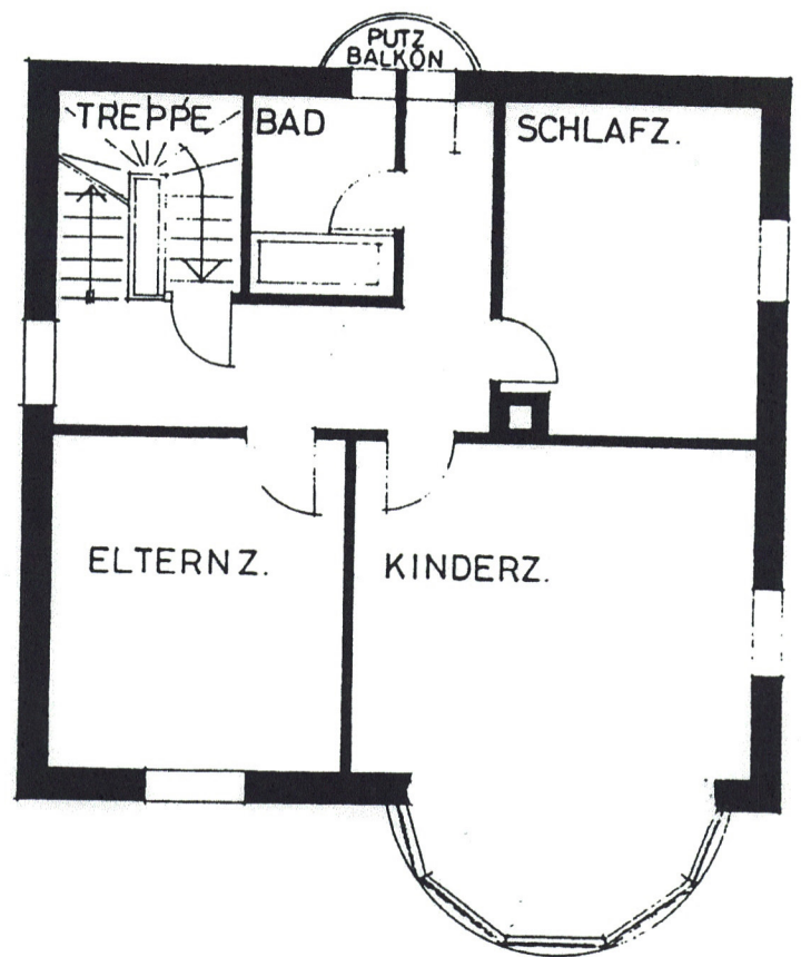
1. OBERGESCHOSS
