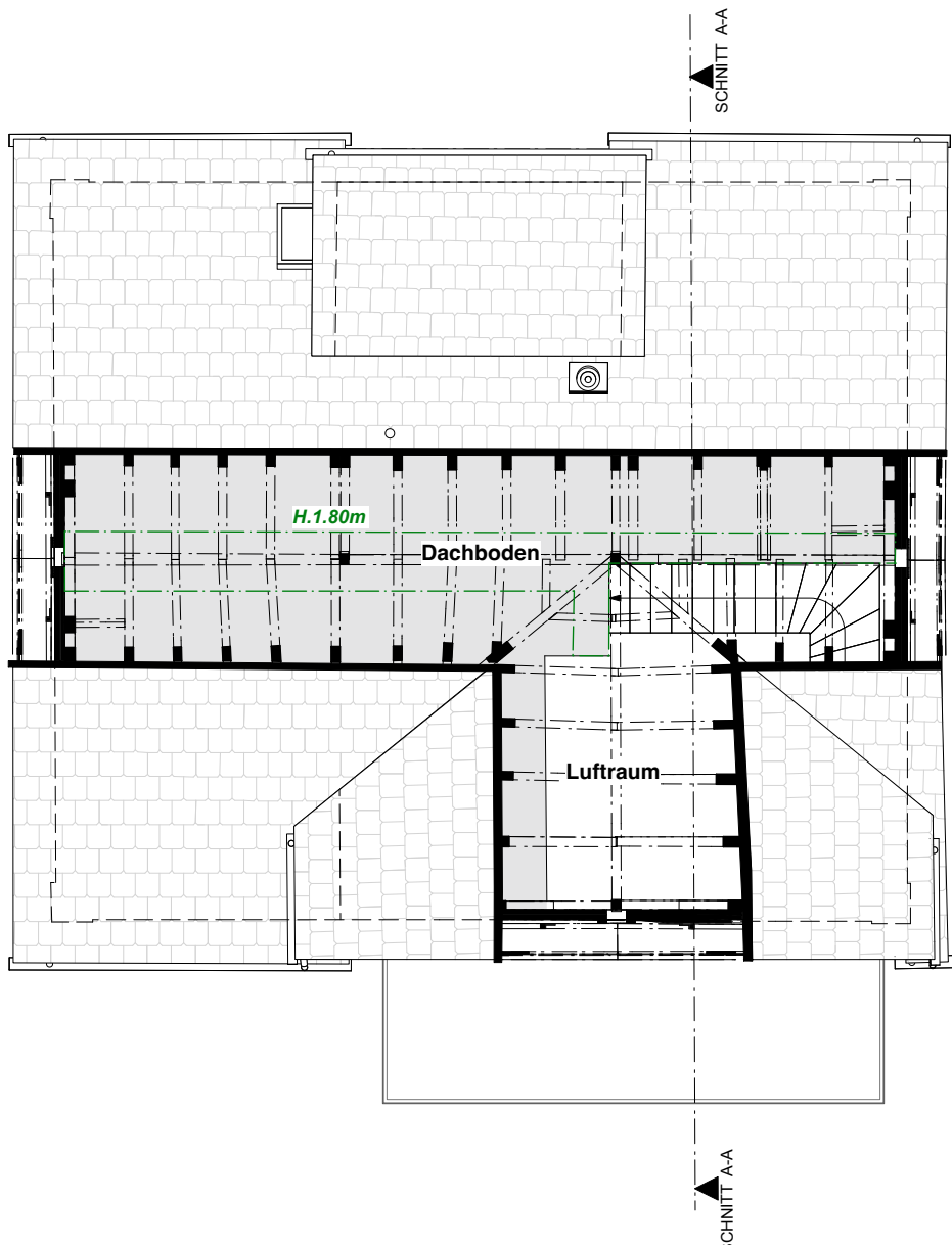
5 Dachboden 1:100
