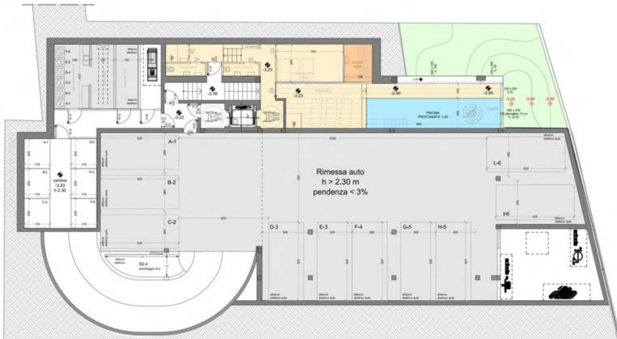
PIANO SEMINTERRATO / INTERRATO
