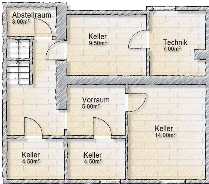
Untergeschoss
