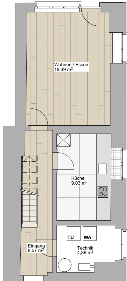
ERDGESCHOSS MST 1:100
