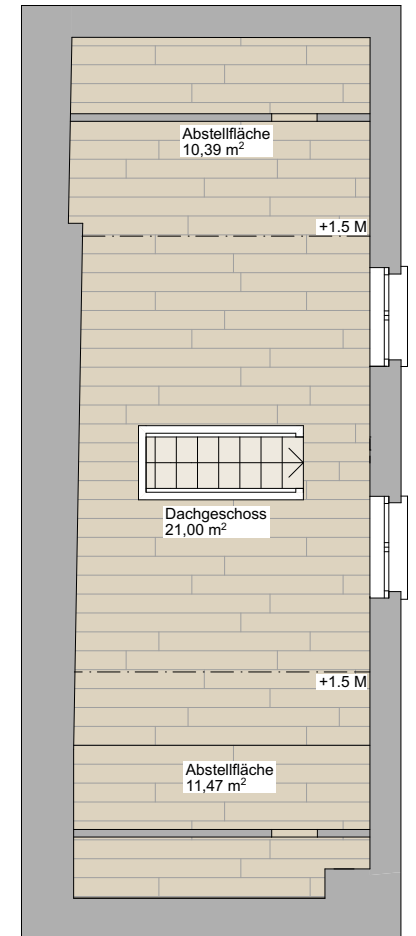
DACHGESCHOSS MST 1:100
