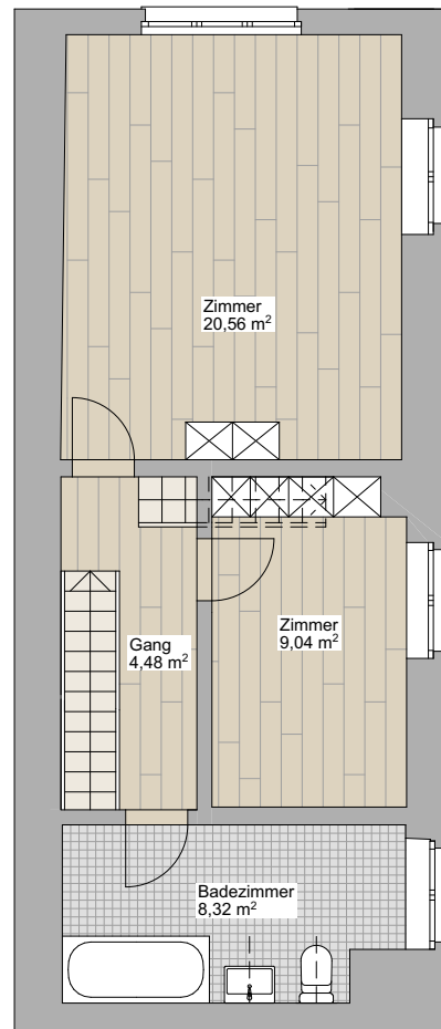
OBERGESCHOSS MST 1:100
