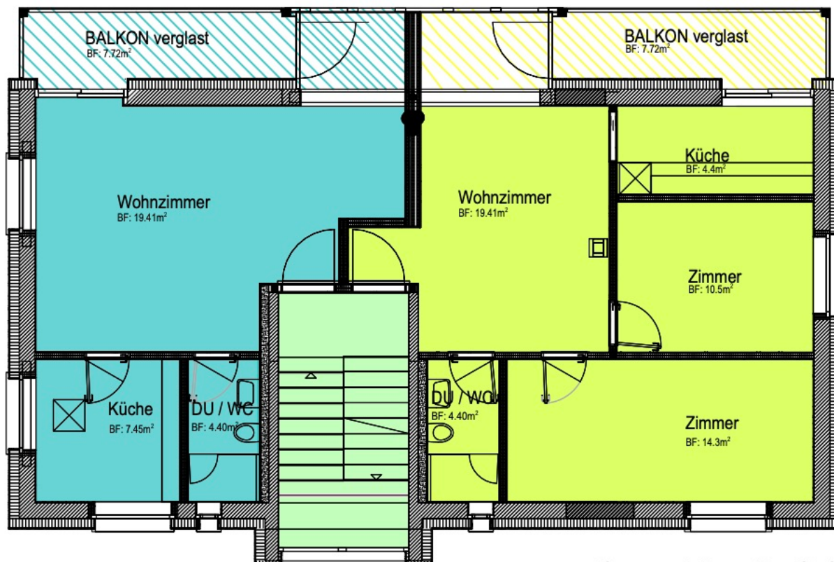
Grundriss 2. OG
