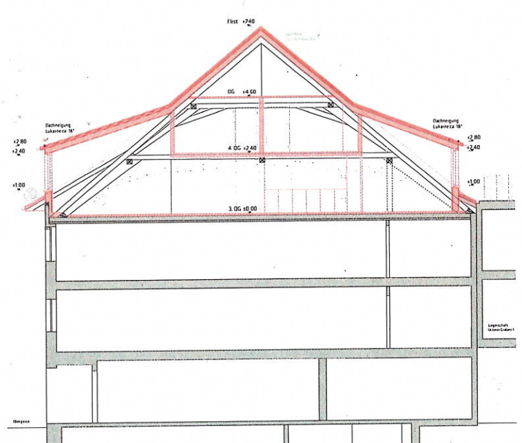
Schema Schnitt
