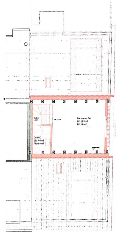
Dachgeschoss
