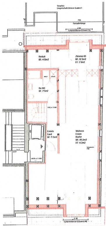
3. Obergeschoss
