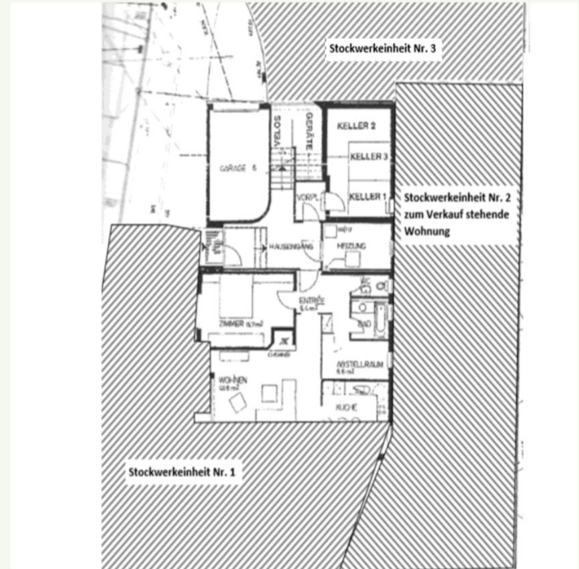
Aufteilungsplan Aussenflächen
