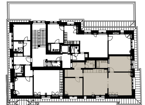
3. Obergeschoss 1:500
