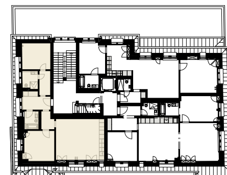
3. Obergeschoss 1:500
