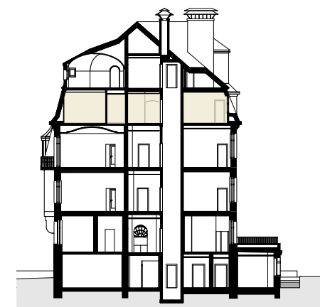
Querschnitt 1:500
