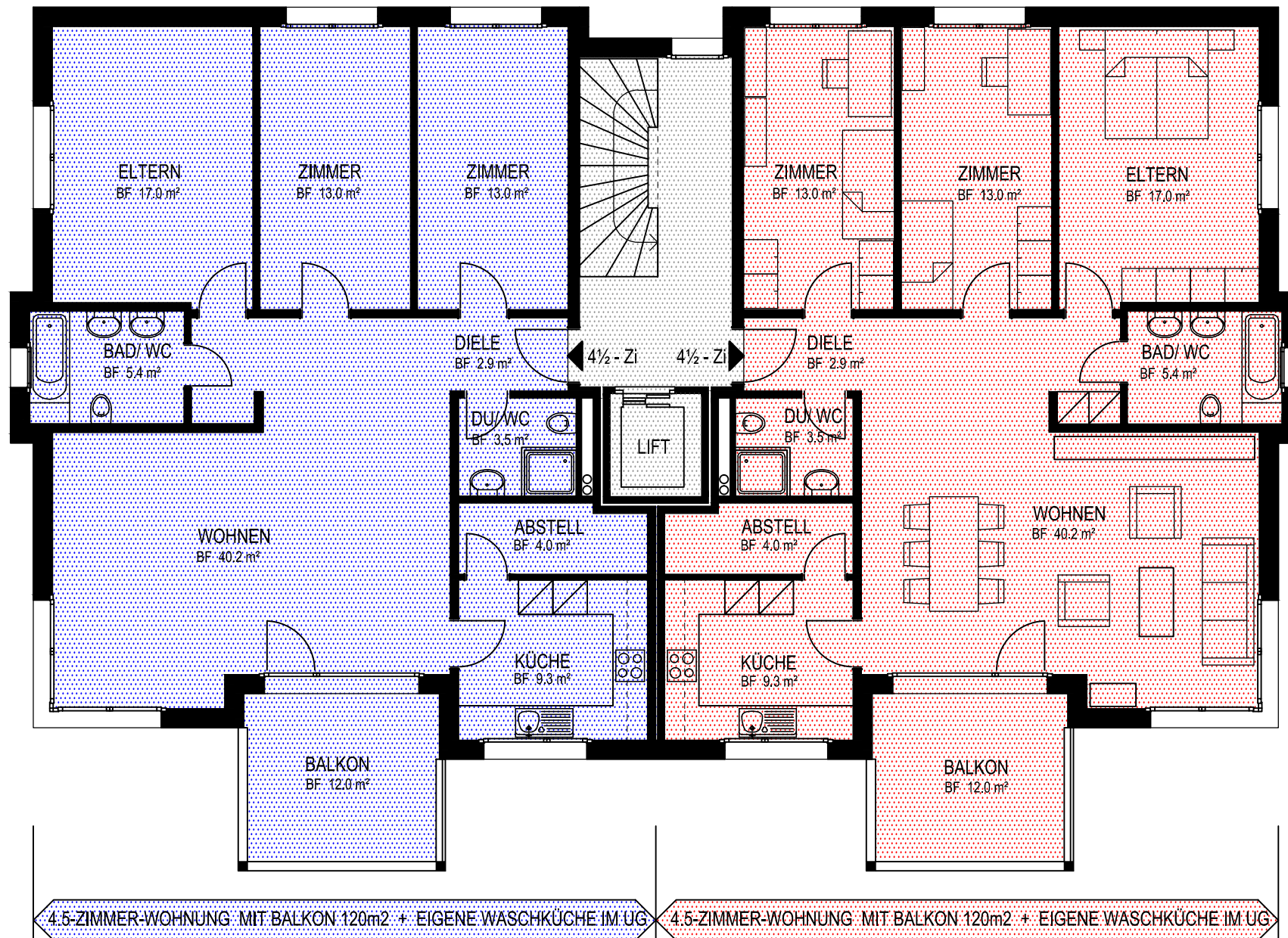
GRUNDRISS OBERGESCHOSS 1:100
