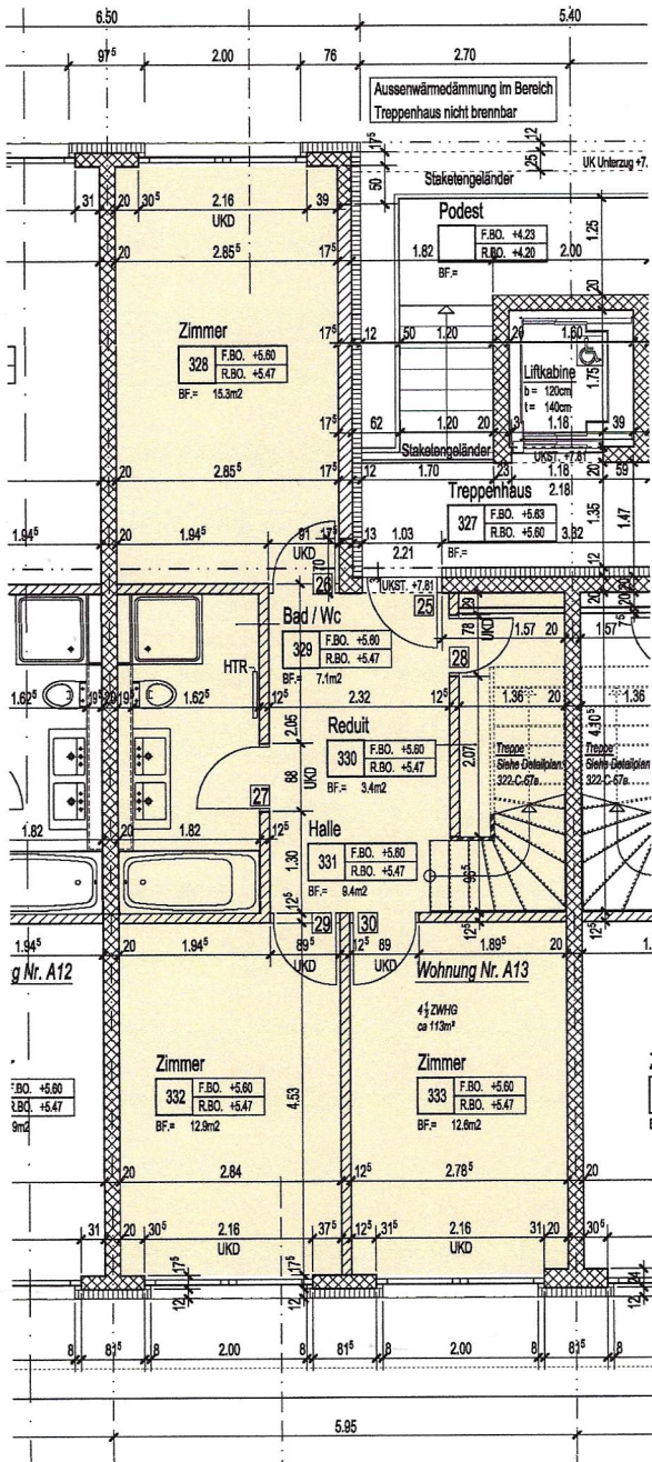
2. Obergeschoss
