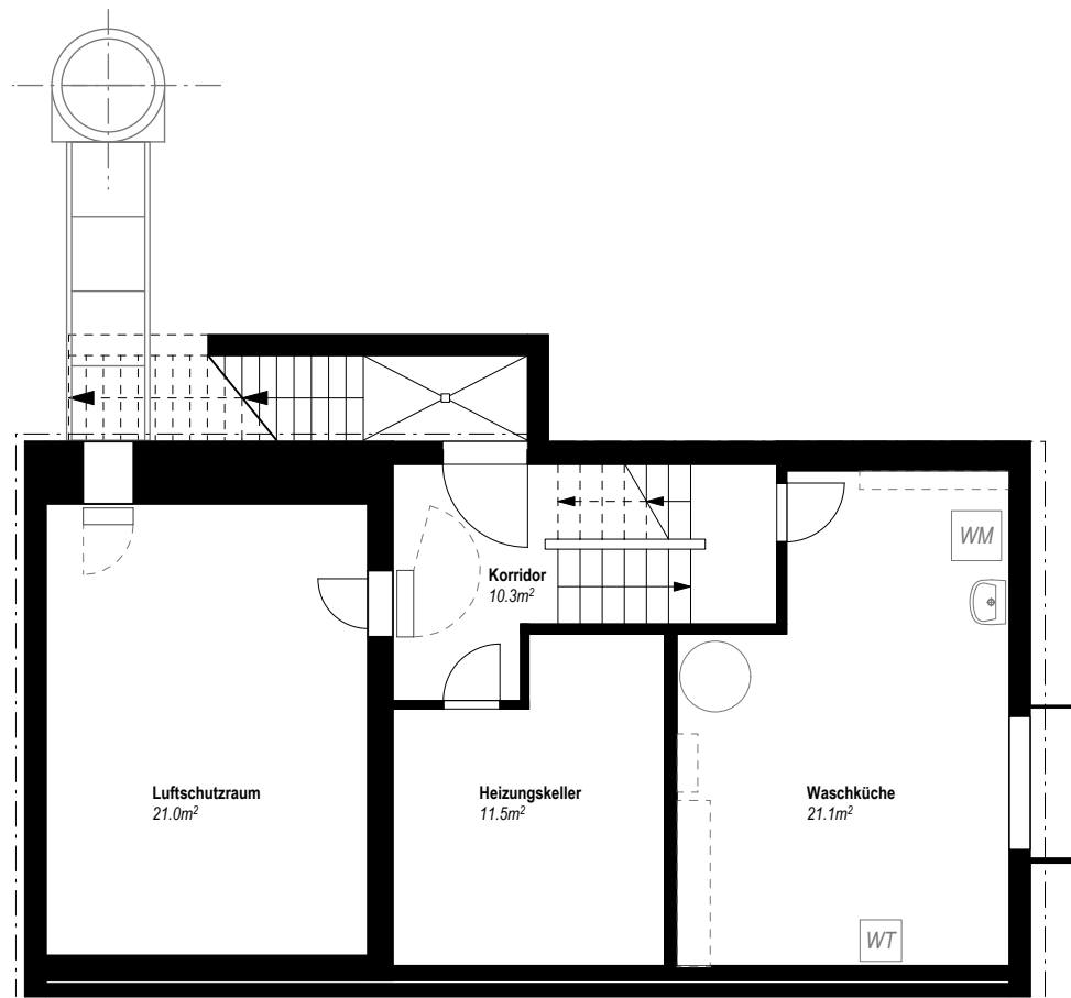
Grundriss Untergeschoss 1:100
