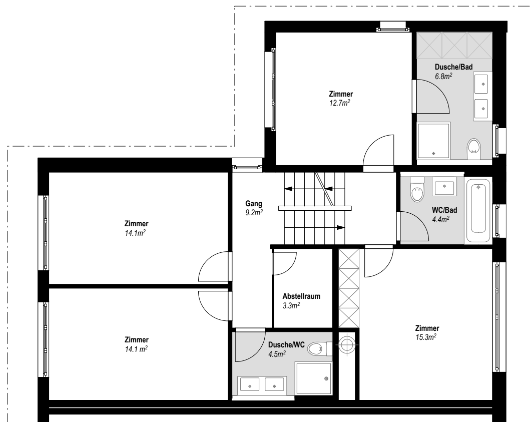
Grundriss Obergeschoss 1:100
