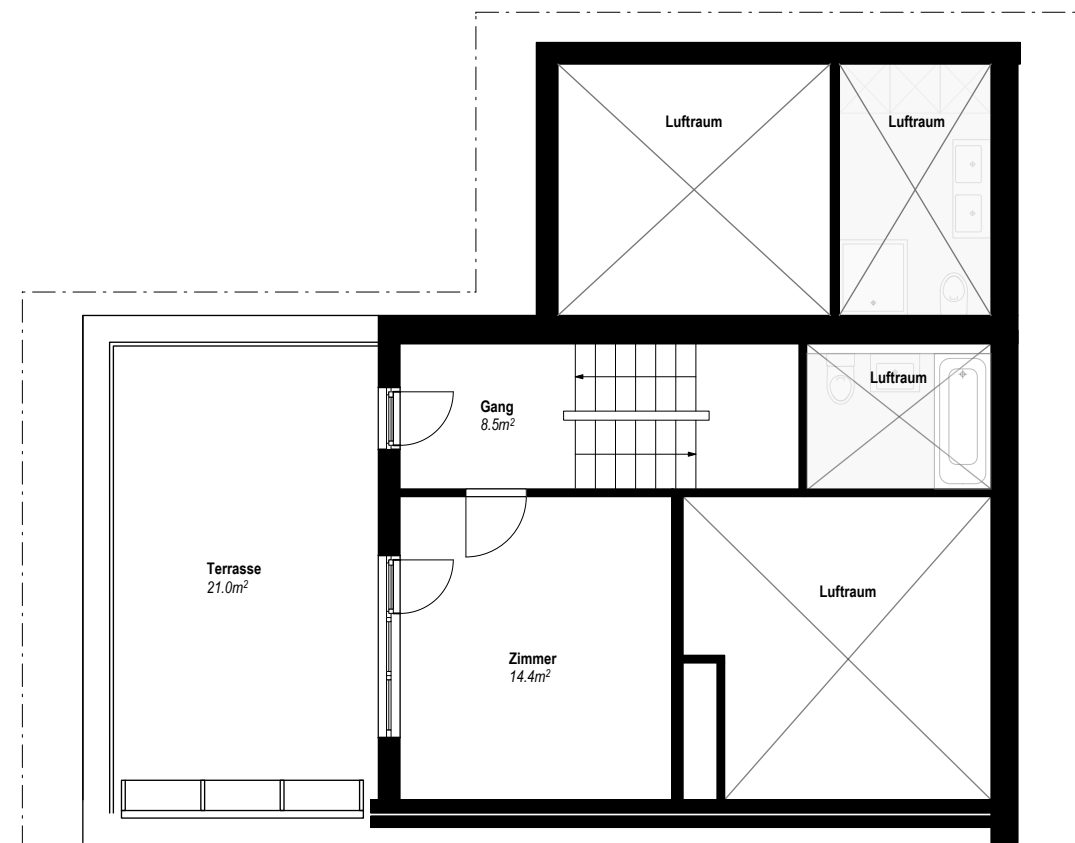
Grundriss Dachgeschoss 1:100
