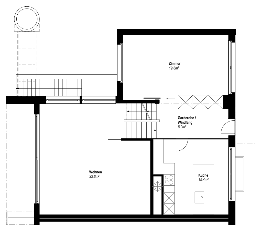
Grundriss Erdgeschoss 1:100
