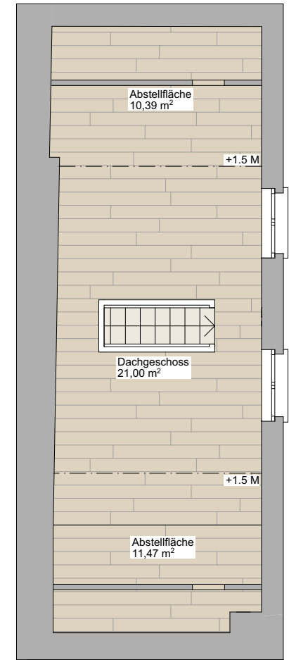
DACHGESCHOSS MST 1:100
