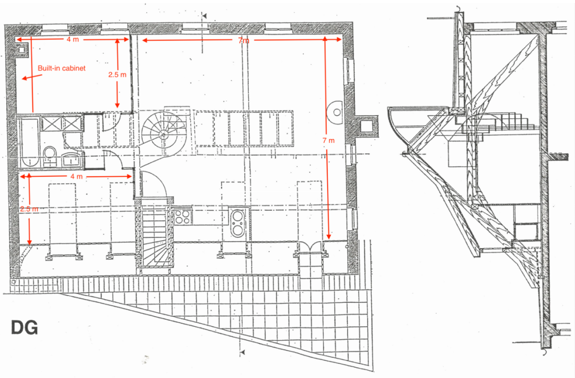
Grundriss der Wohnung
