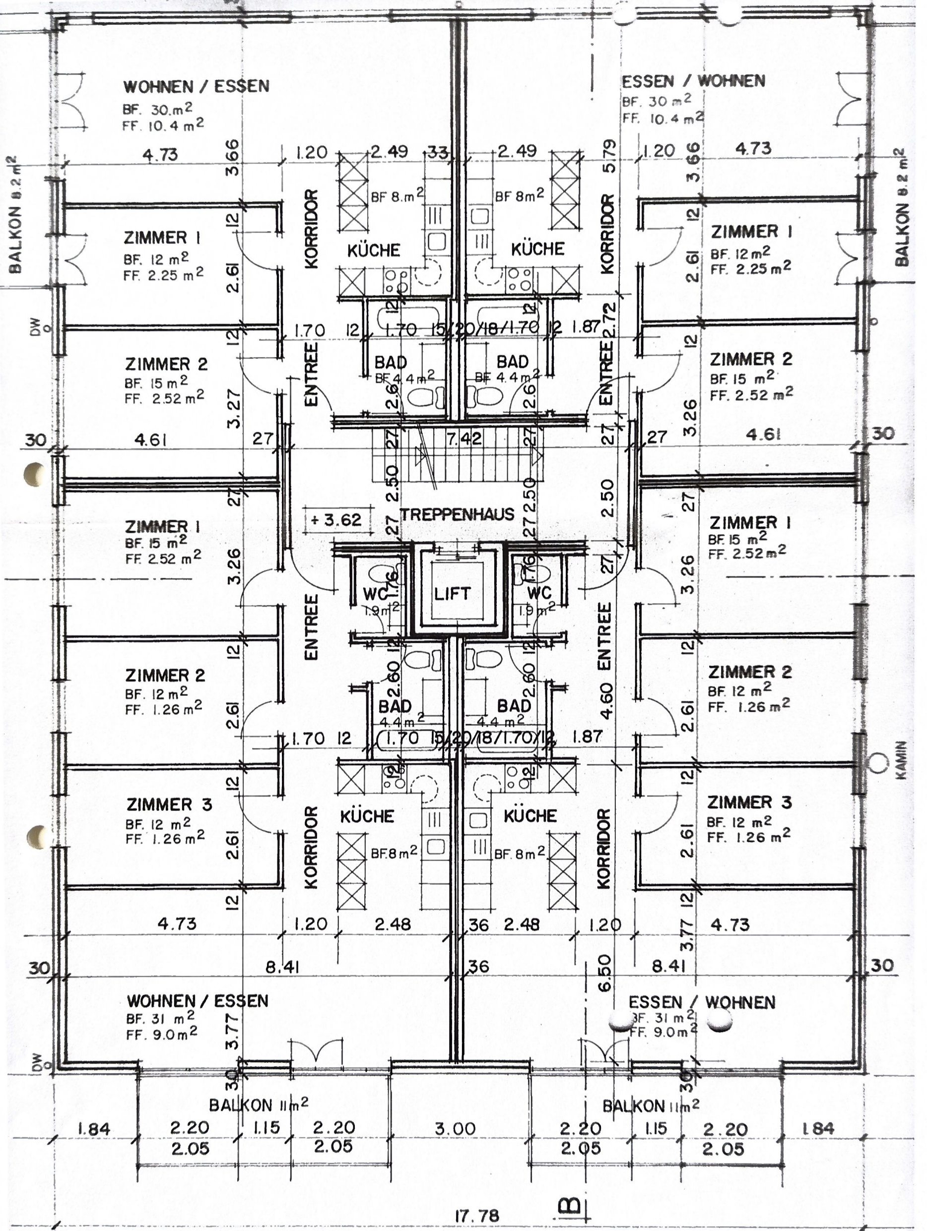
GRUNDRISS 1. OBERGESCHOSS
