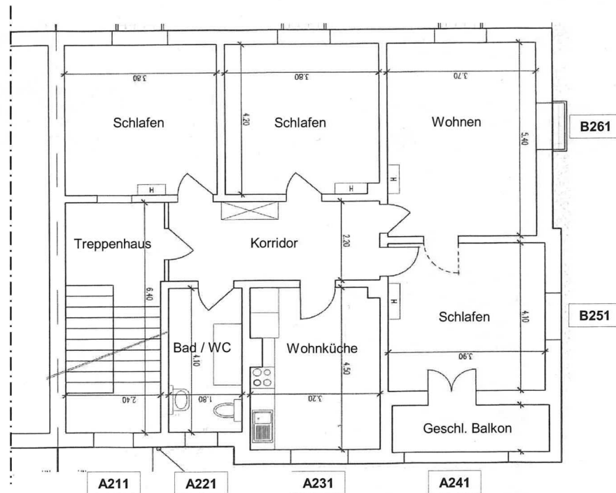
Grundriss 2. Obergeschoss
