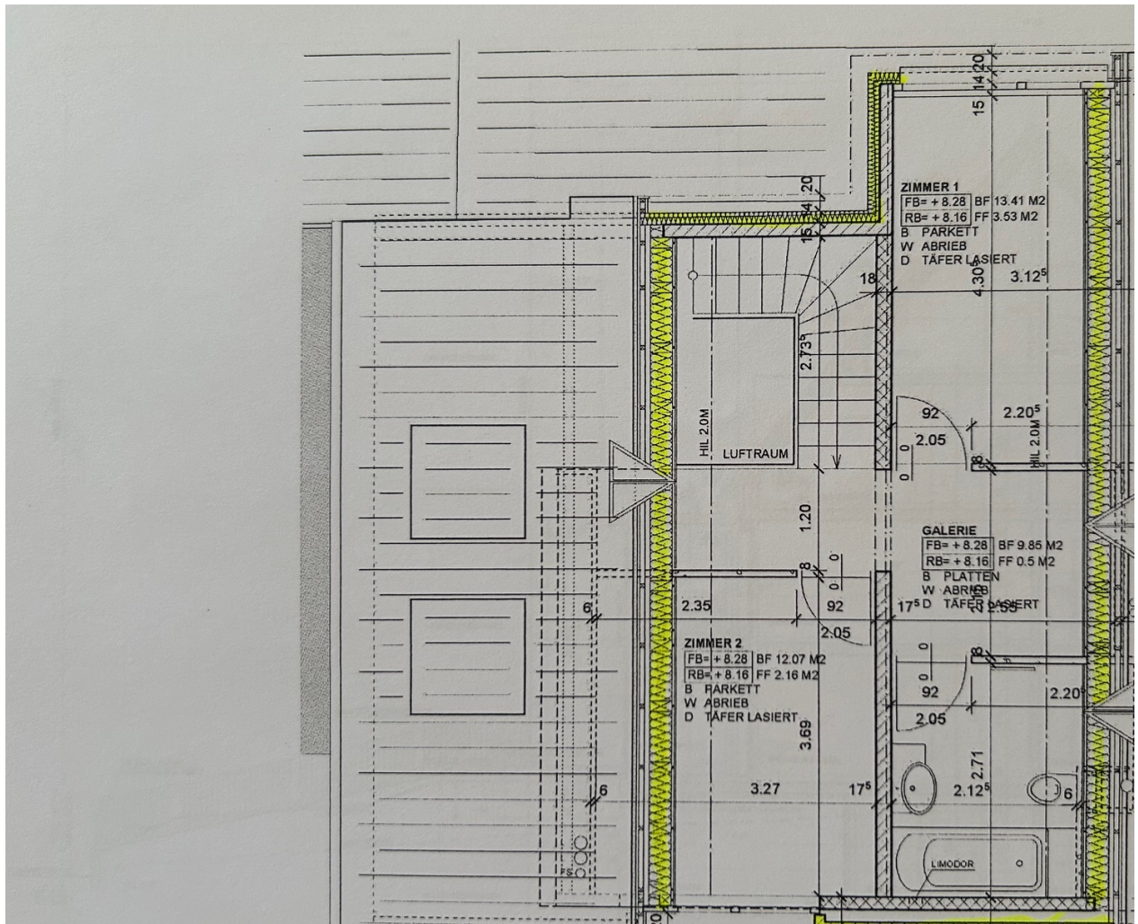
Dachgeschoss
