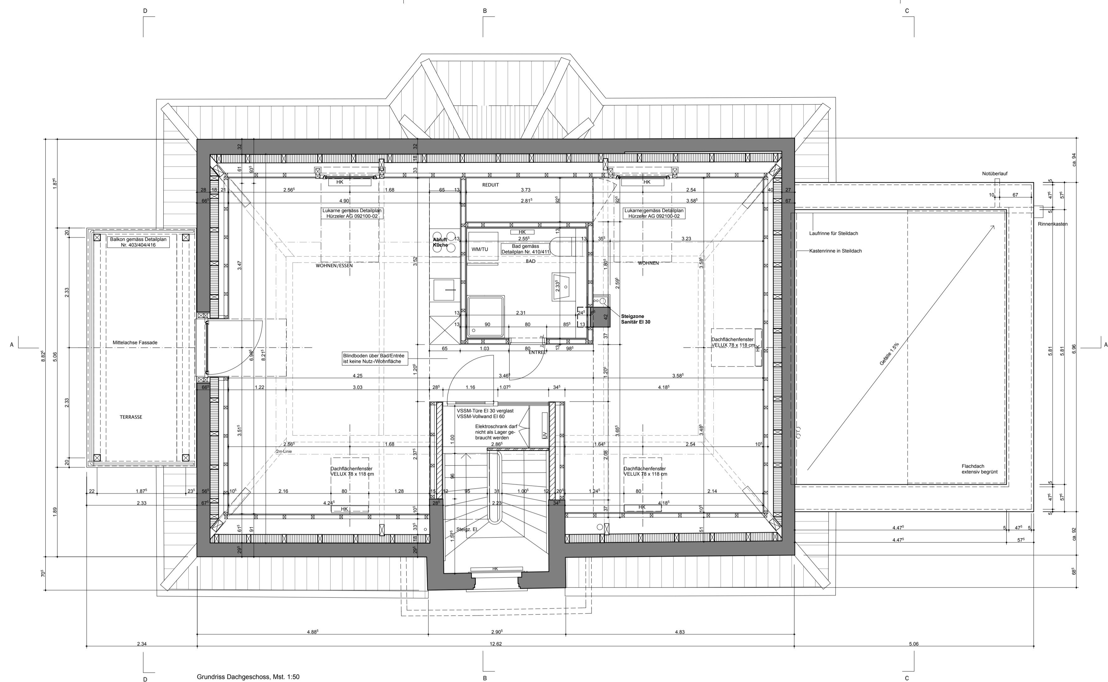
Grundriss Dachgeschoss, Mst. 1:50
