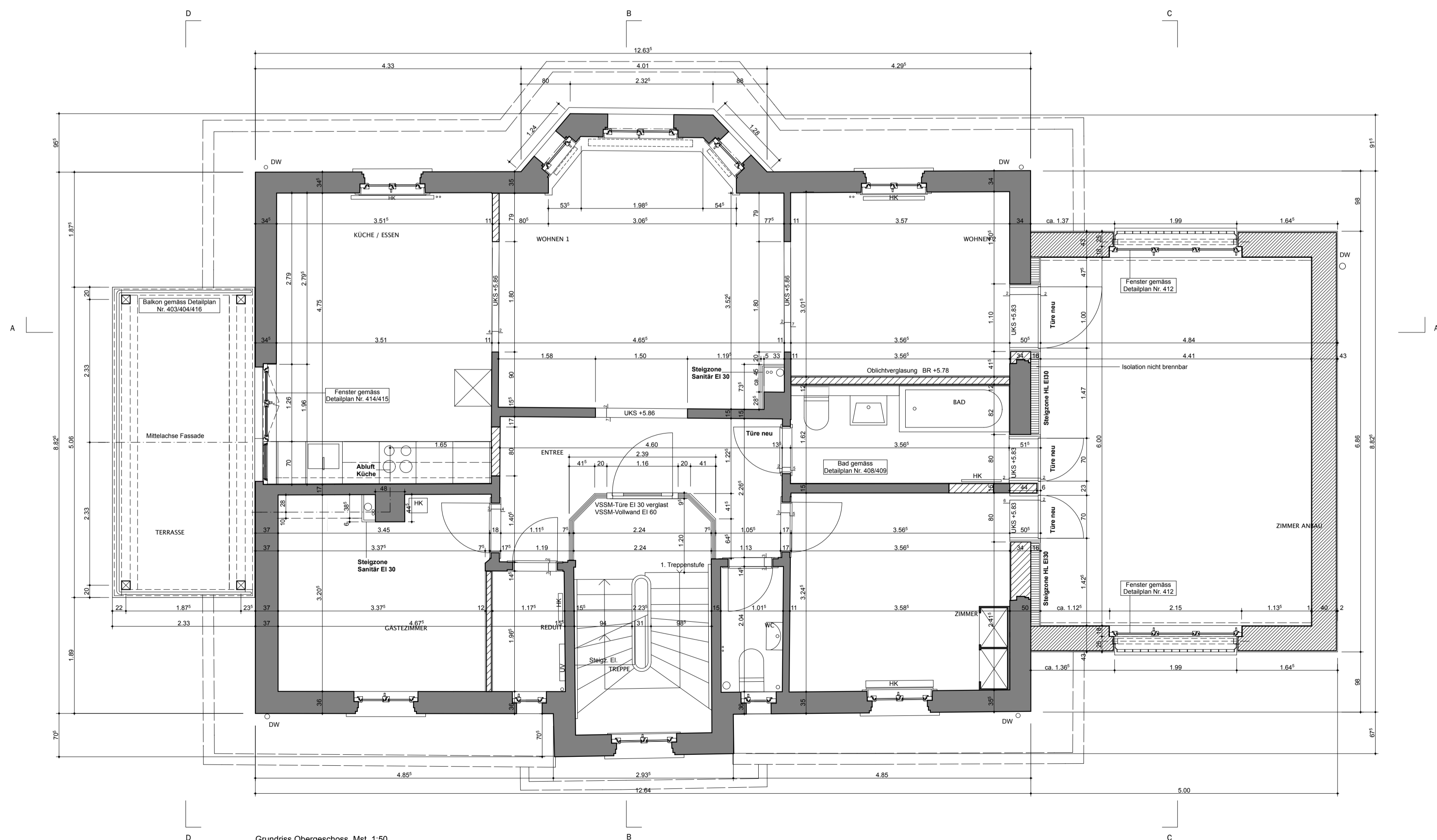
Grundriss Obergeschoss, Mst. 1:50
