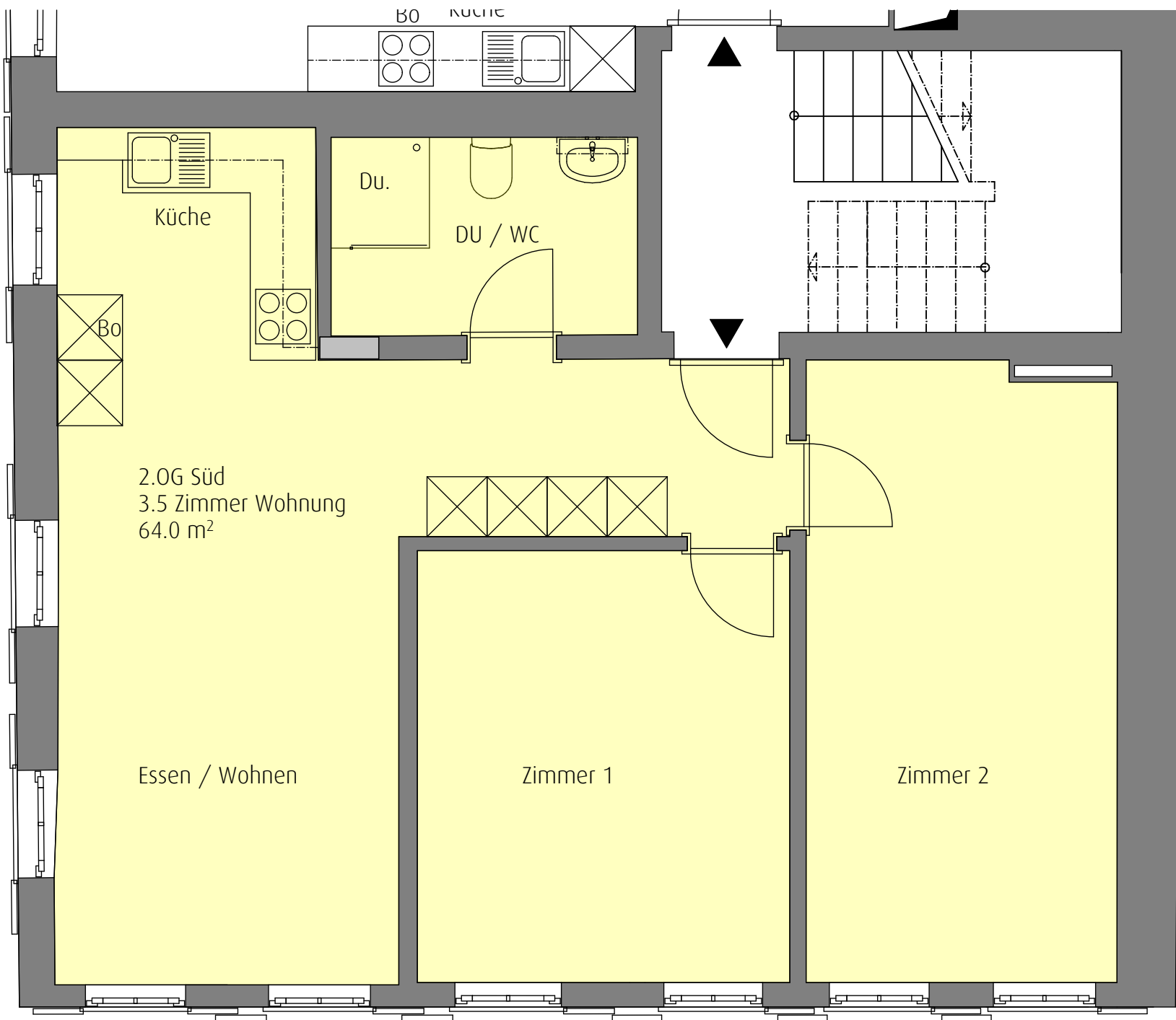
Grundriss 2. OG Süd 3.5 Zimmer Wohnung
