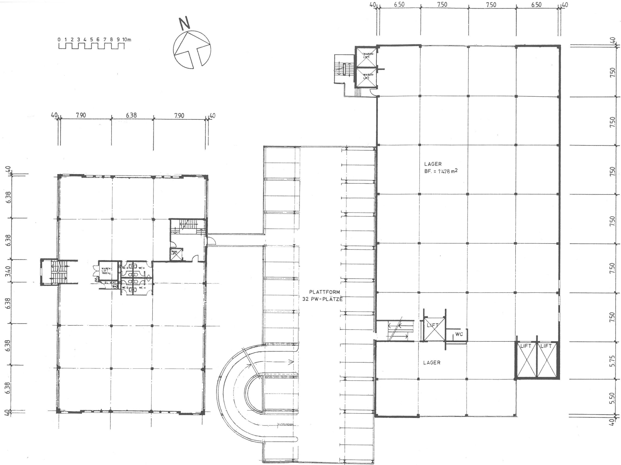
BÜROGEBÄUDE 2., 3.+4.OG / 2.+3. PARKDECK/LAGERGEBÄUDE 1.+2.OG
