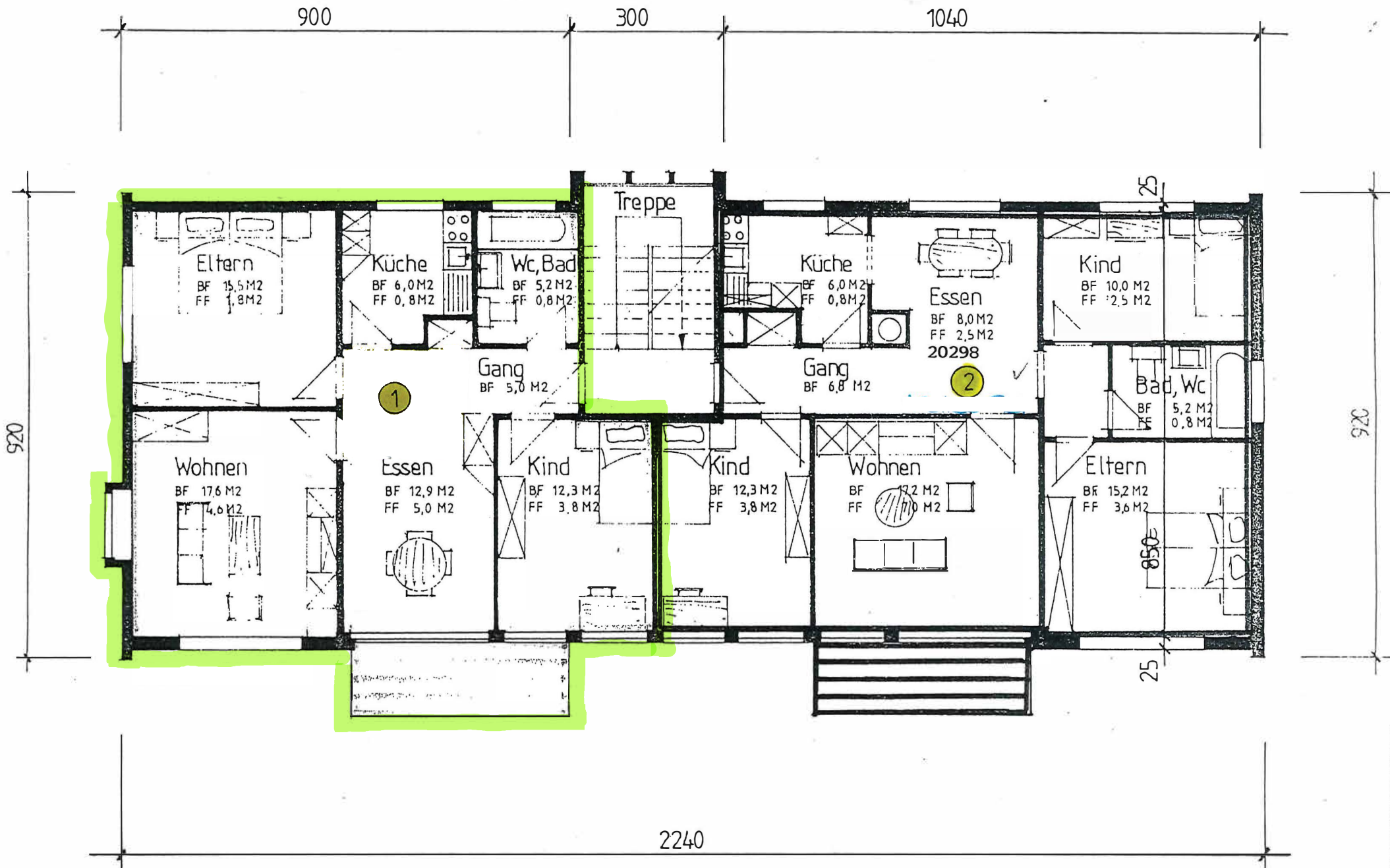
Grundriss 1:100
