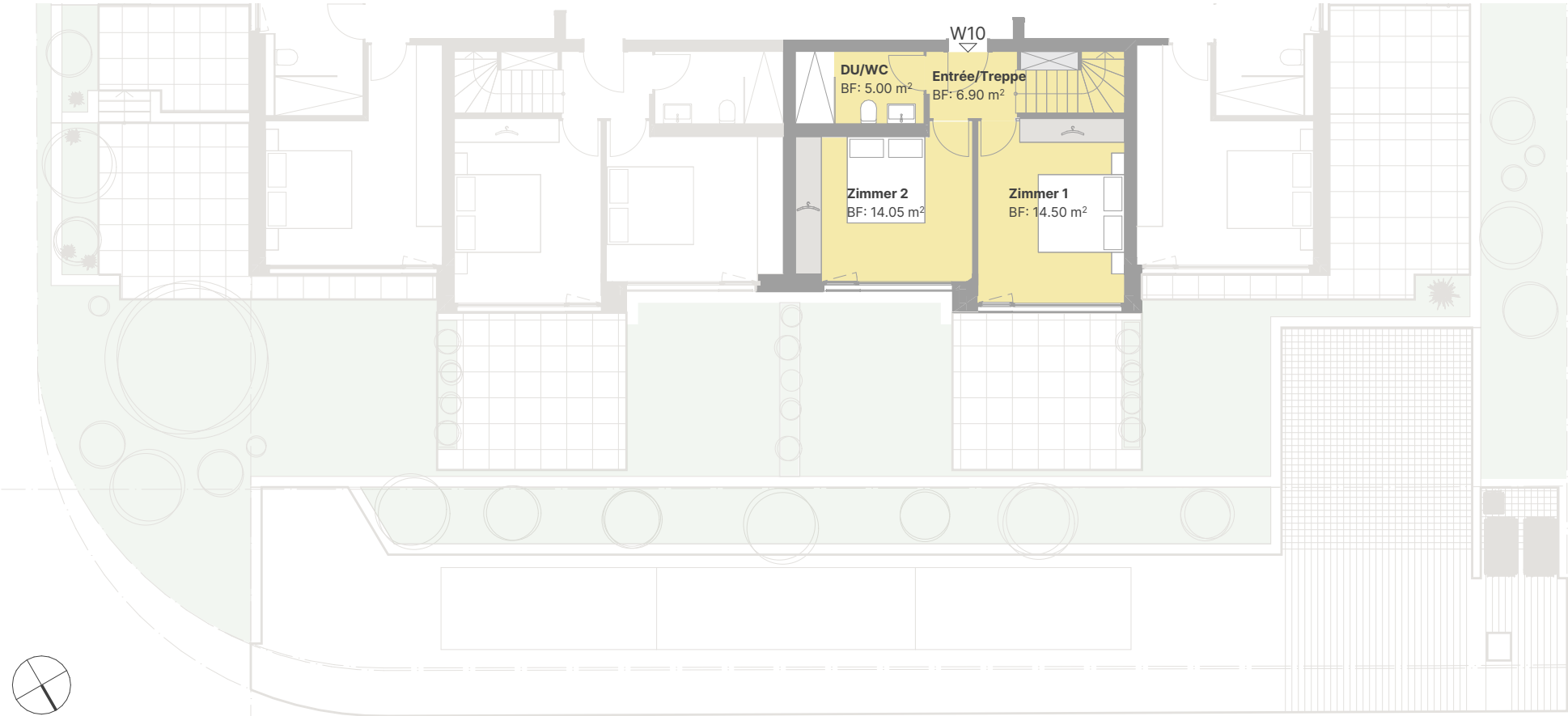
Erdgeschoss
