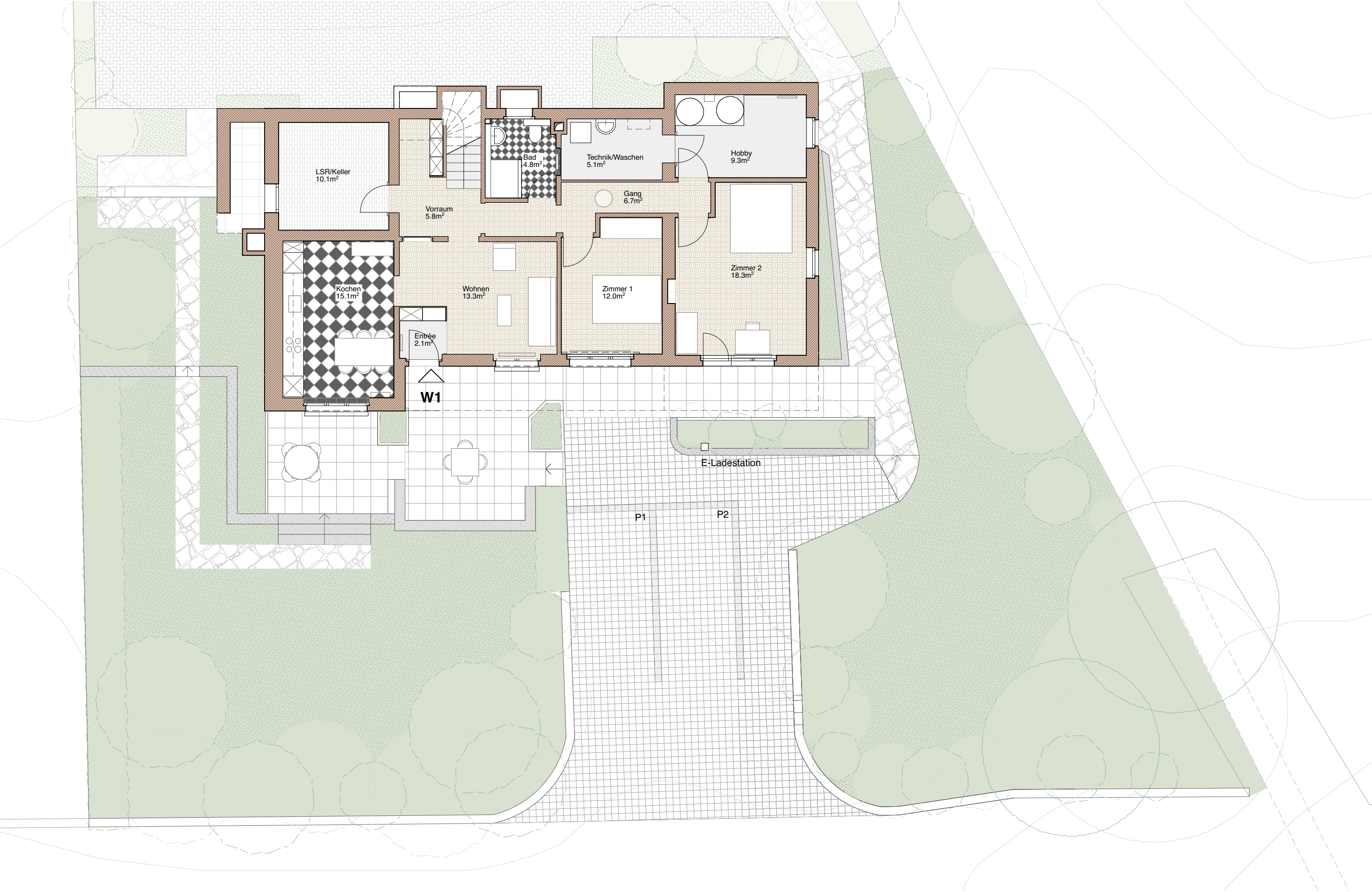
ERDGESCHOSS 1:100 | WOHNUNG 1
