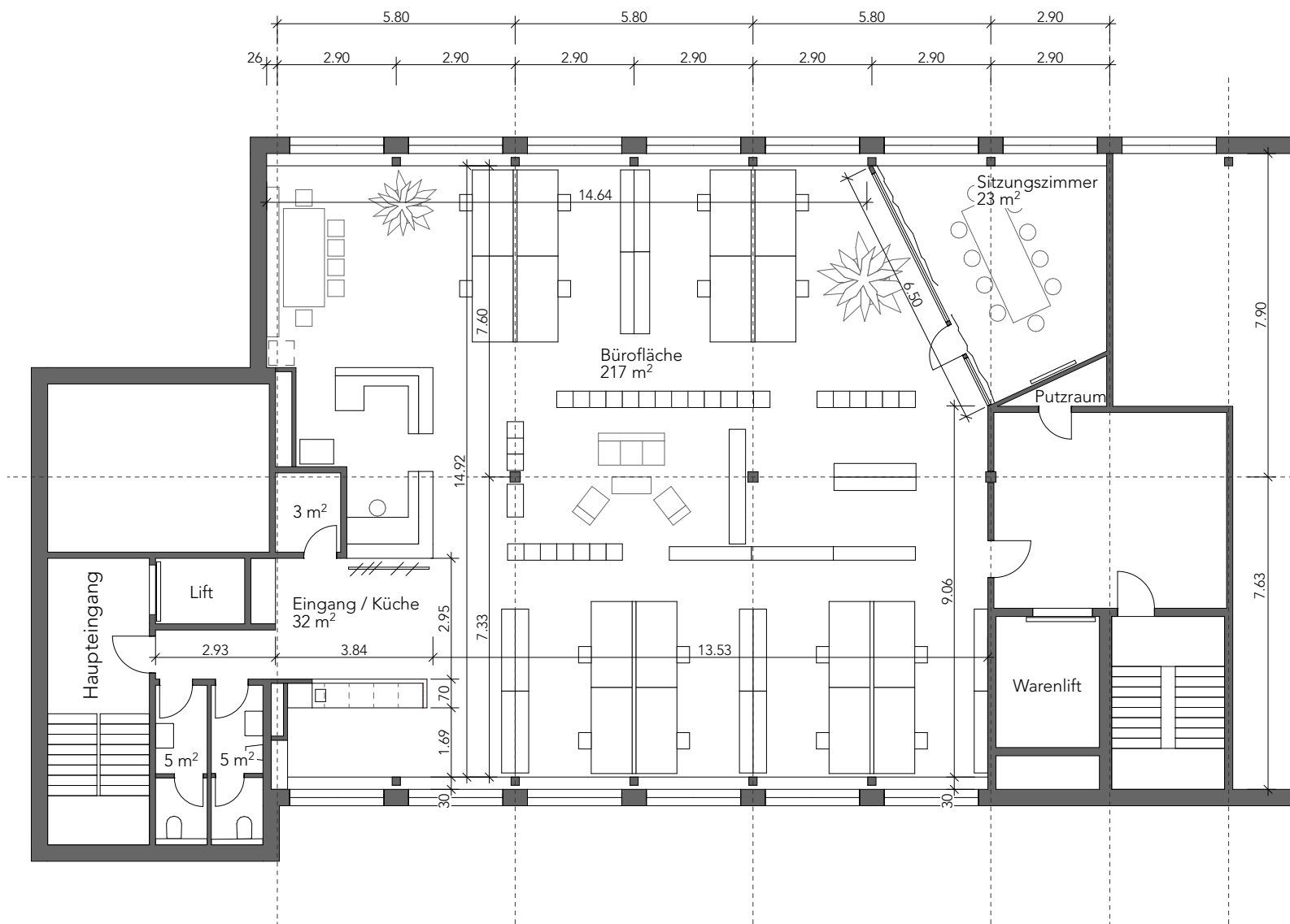
Grundriss OG4
