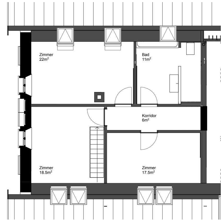
Grundriss Dachgeschoss 1:100
