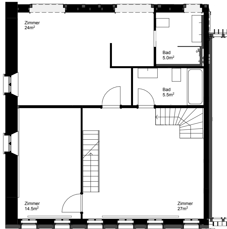
Grundriss Erdgeschoss 1:100
