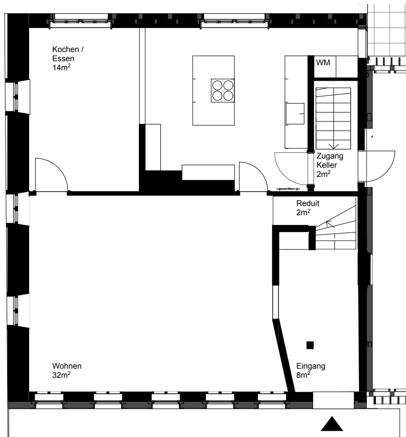
Grundriss Erdgeschoss 1:100
