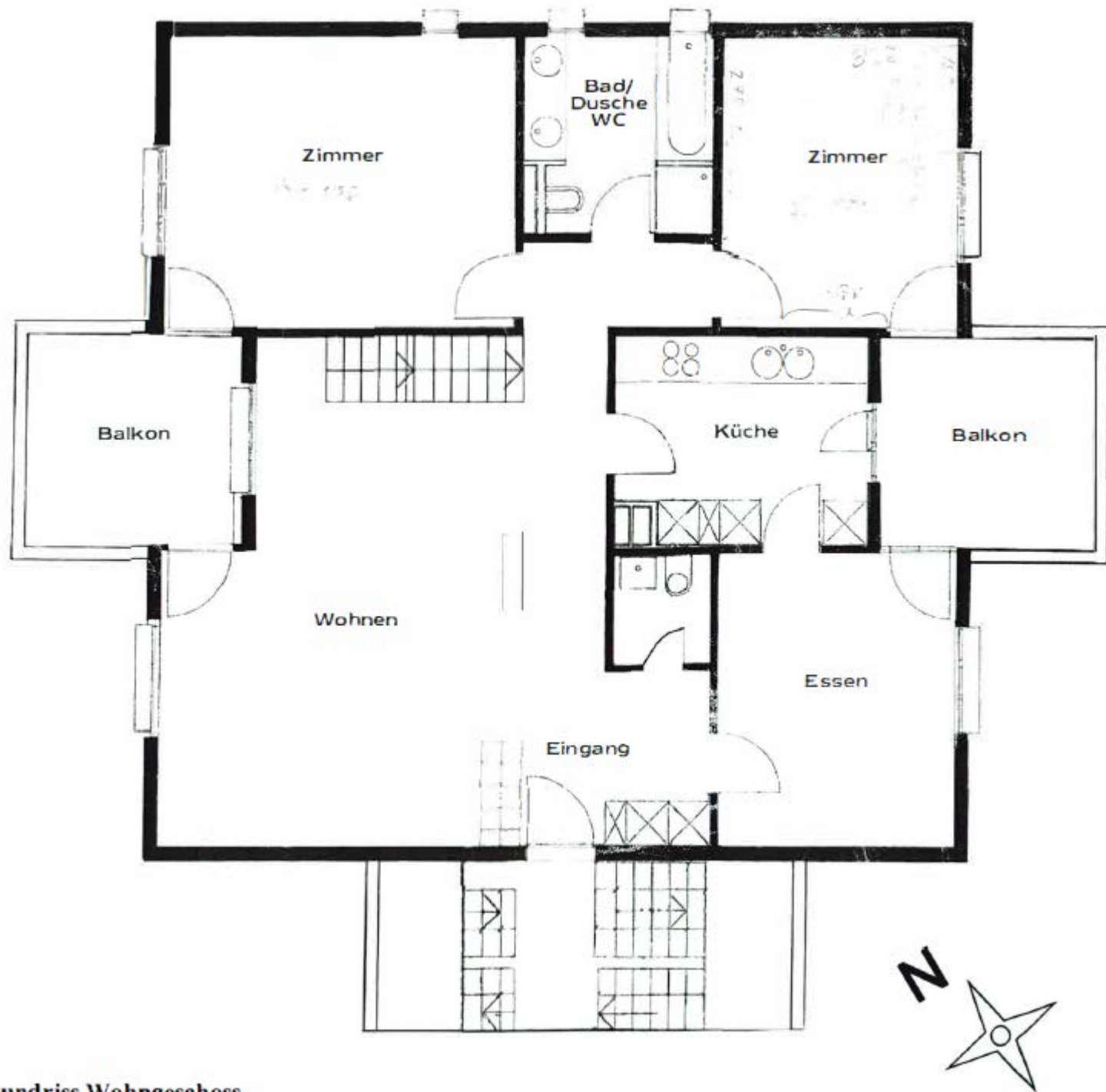
Grundriss Wohngeschoss
