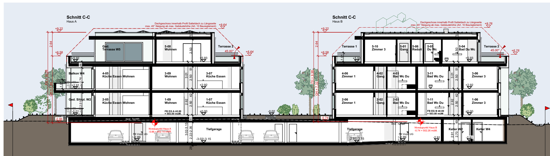
SNITT C-C
