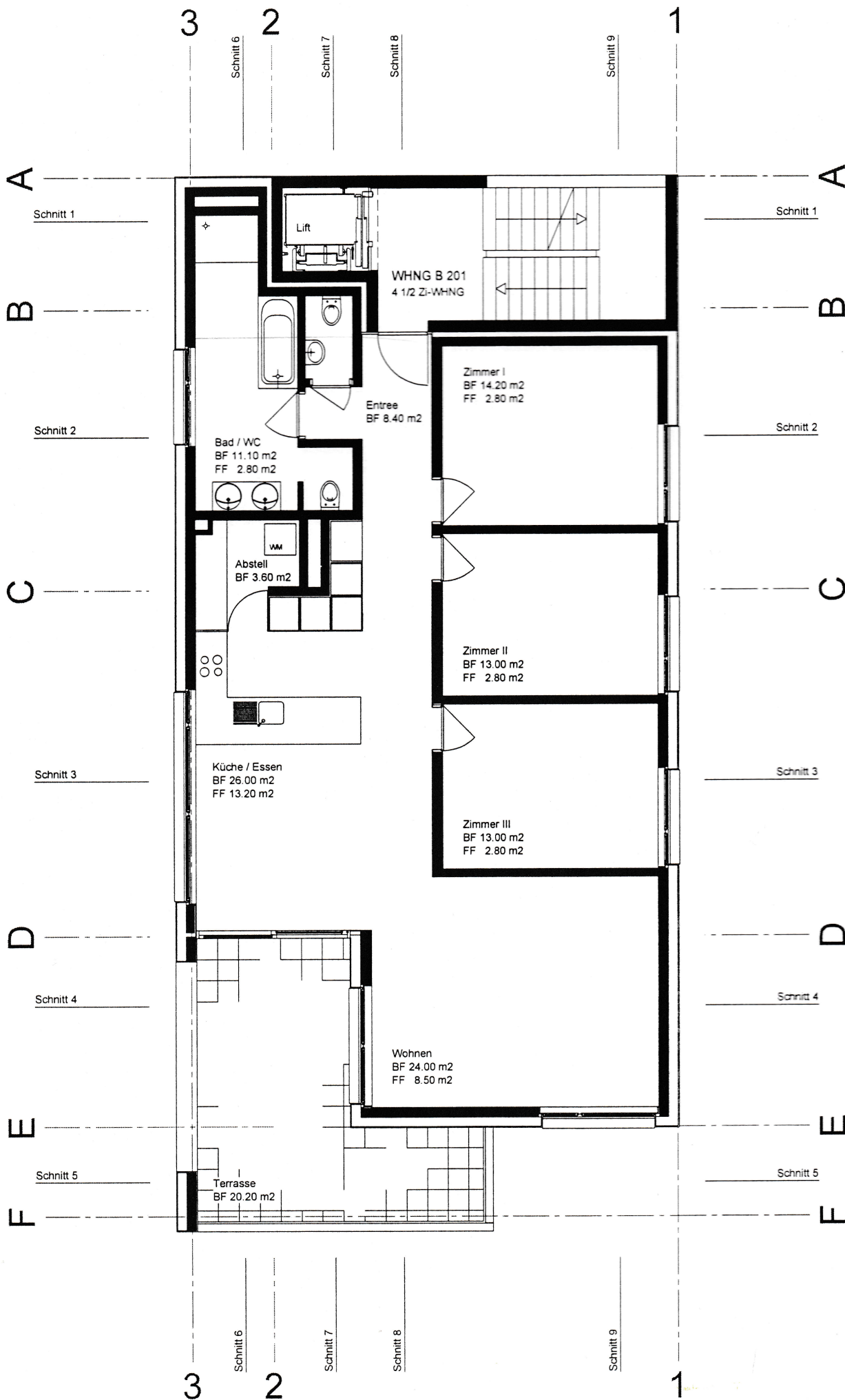
2.Obergeschoss 1:100
