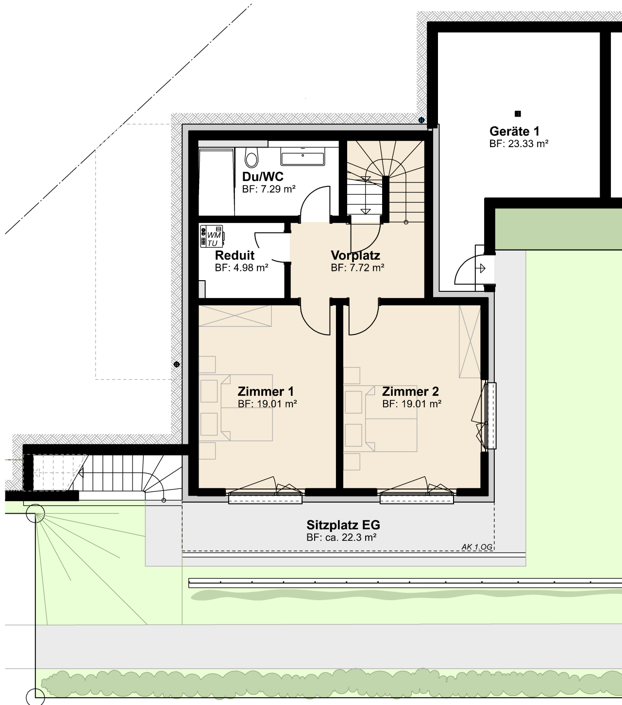
Grundriss Erdgeschoss
