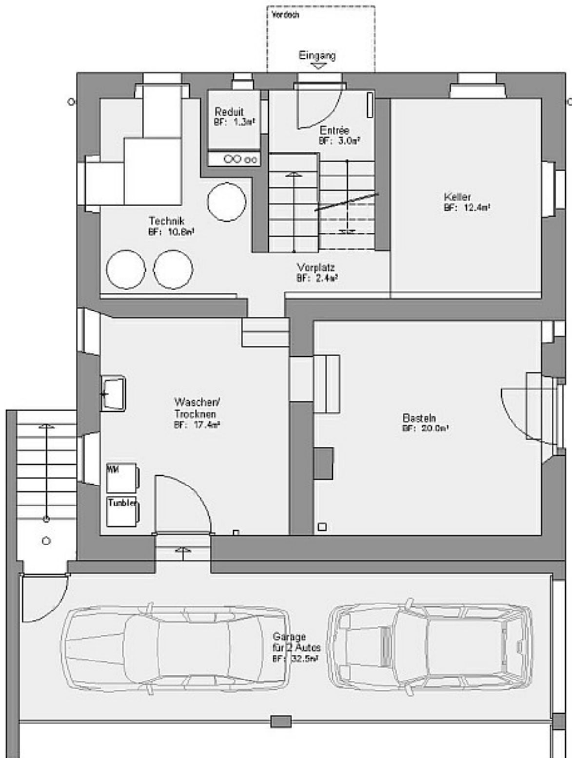
Untergeschoss 0 0.5 1 2 2m
