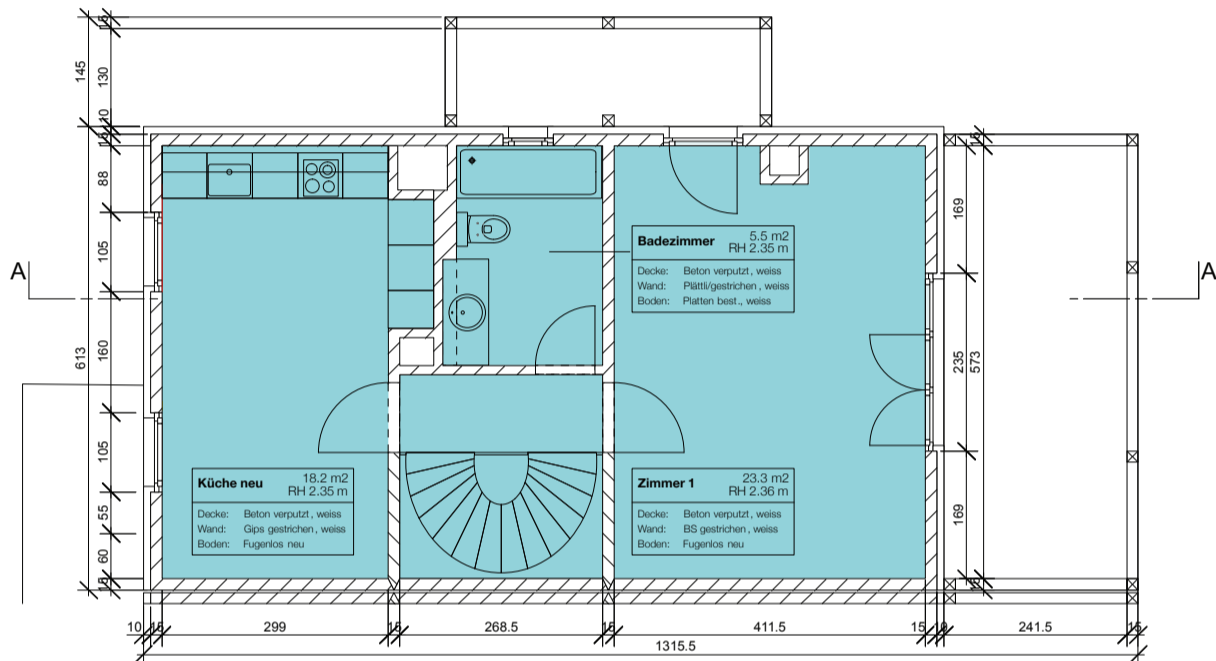
OBERGESCHOSS
