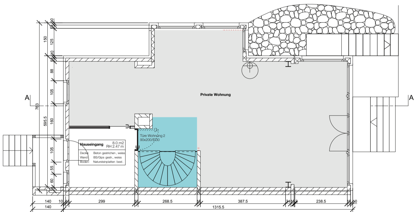
ERDGESCHOSS
