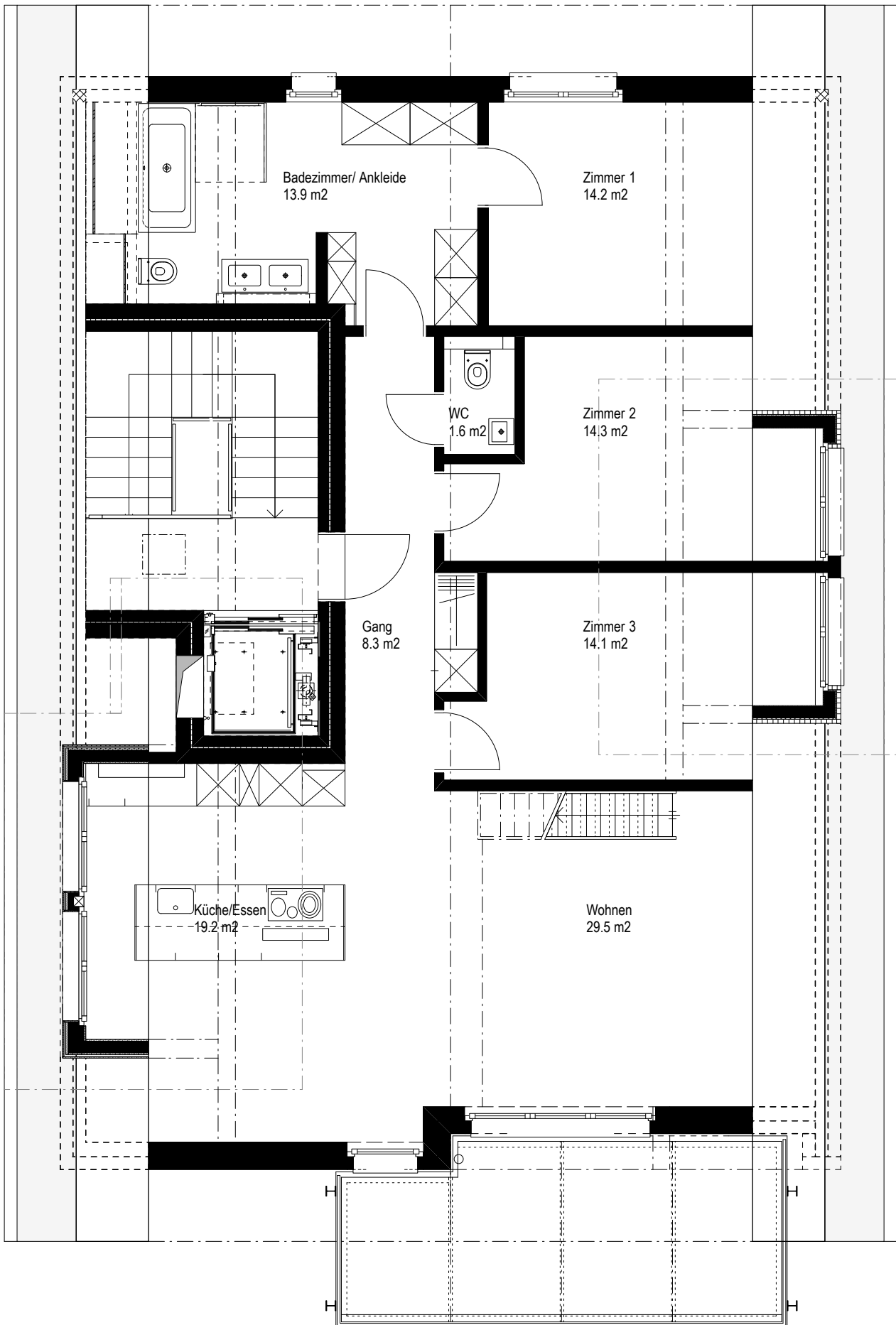
Dachgeschoss
