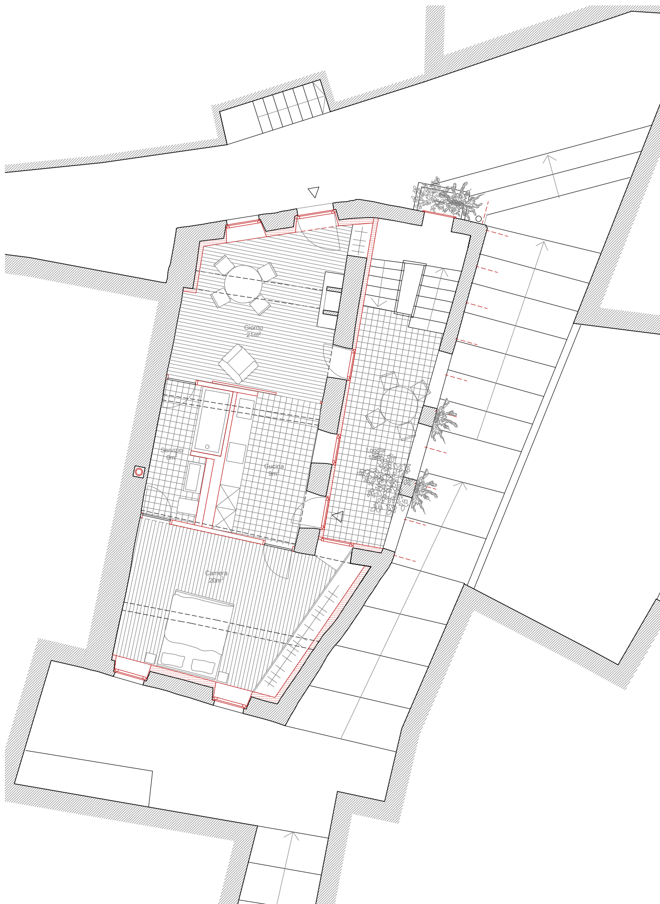
Primo Piano Variante per 2 unità appartamento separato
