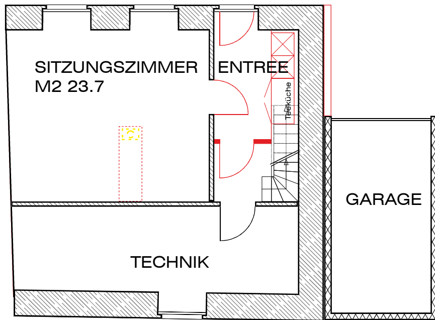
UNTERGESCHOSS
