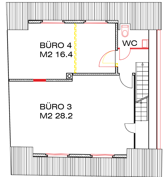
DACHGESCHOSS
