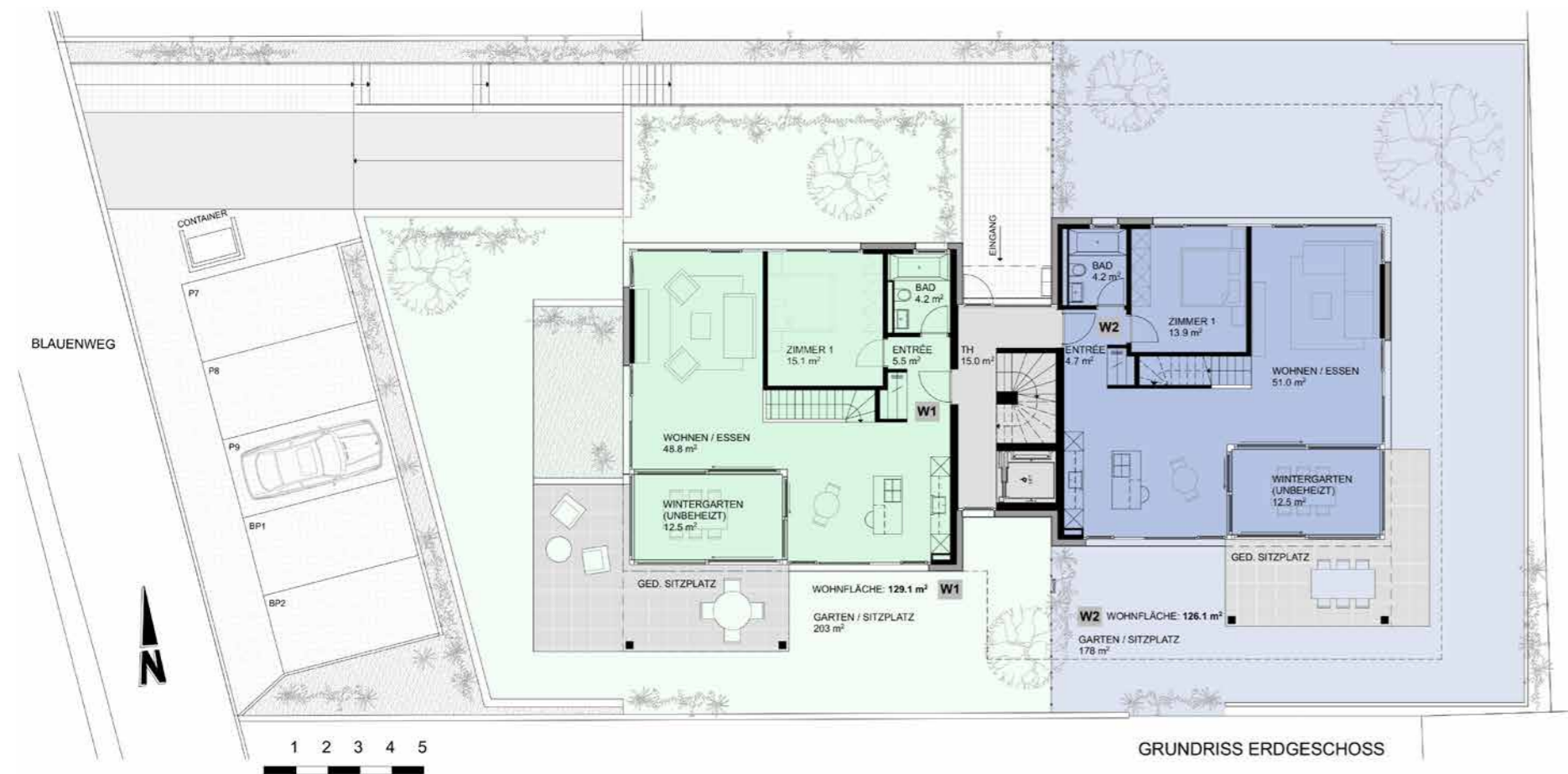
Maisonette - Wohnung W1 4.5 Zimmer = 130.3 m 2
