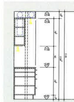
Schnitt Küche
