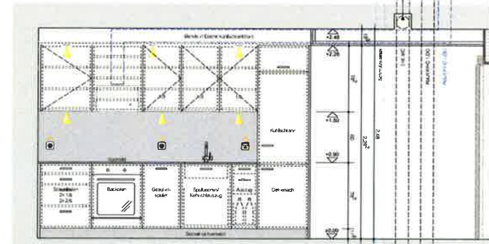
Ansicht Küche
