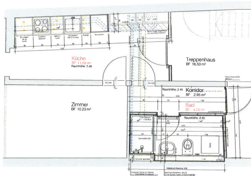
2. Obergeschoss
