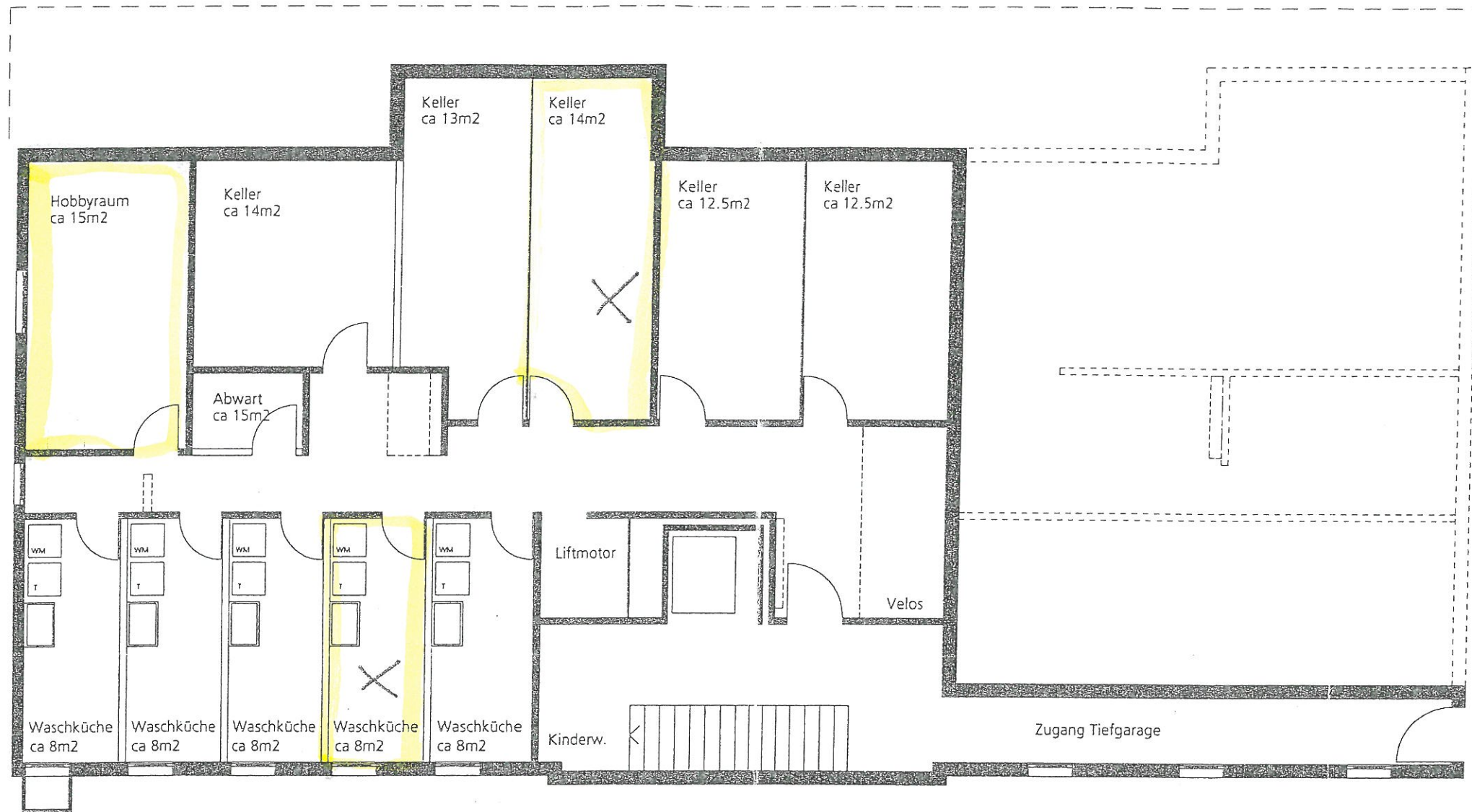
Untergeschoss
